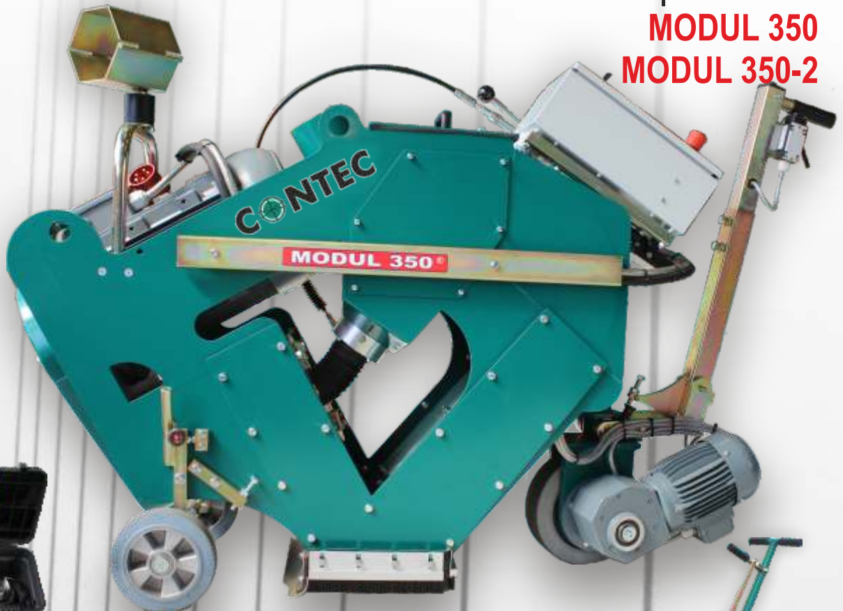
Schleuderrad mit 6 Flügeln blast wheel with 6 blades
